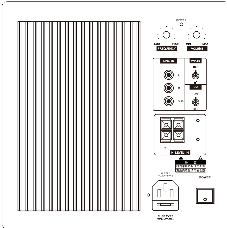
图1 SUB-10B-N 放大器背板示意图
