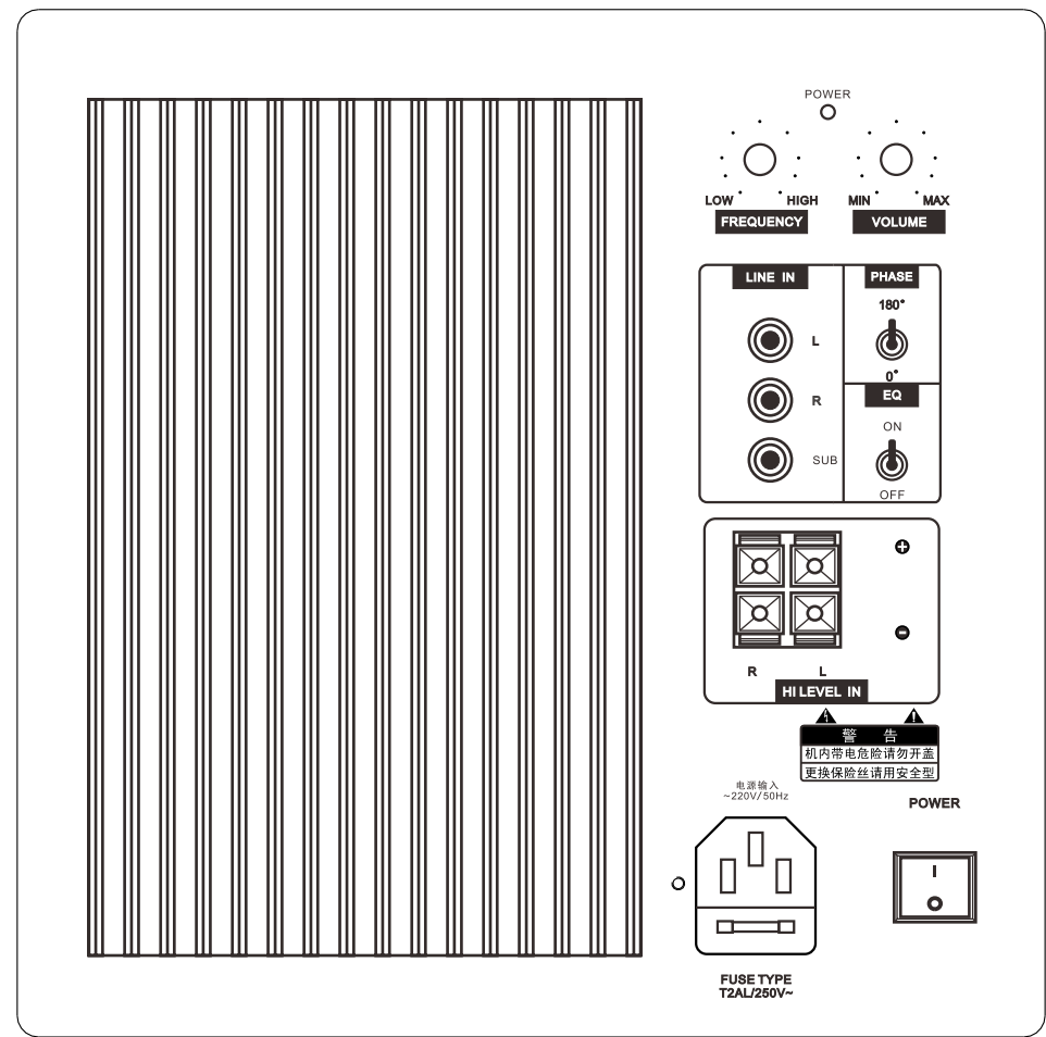
图1 SUB-10PA放大器背板示意图
