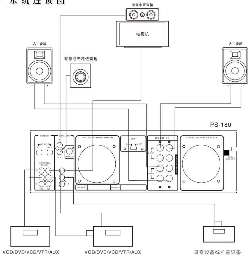
PS-180系统连接示意图
